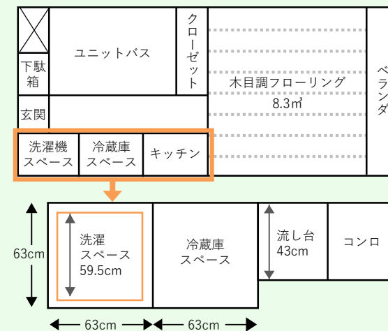
間取り図
